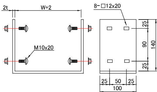
角根丸頭ボルト・ナット 8組合む
