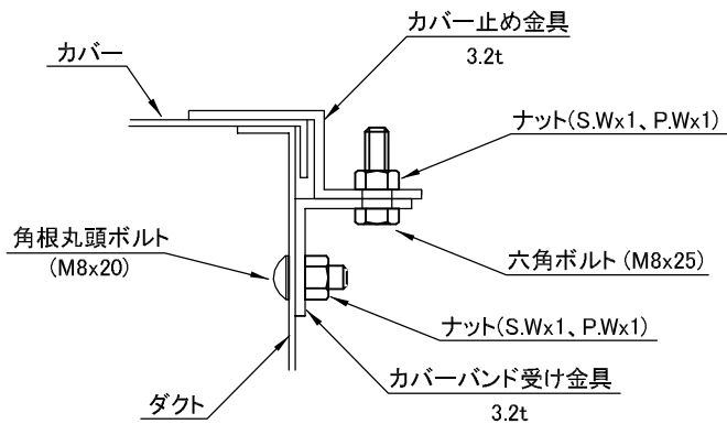
"A"部 詳細仕様
