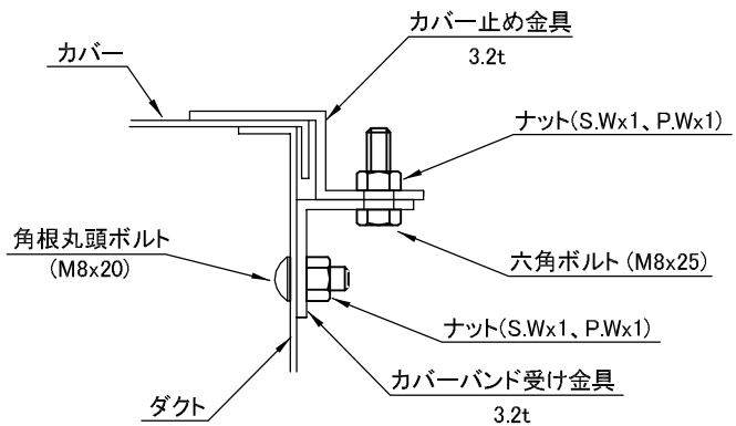
“A”部 詳細仕様
