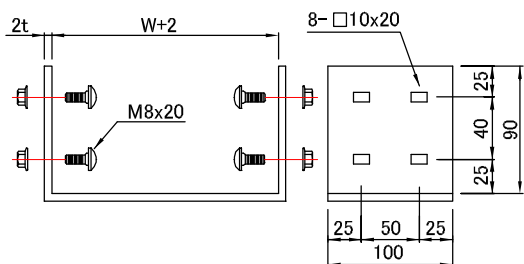
角根丸頭ボルト・ナット 8組合む
