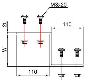
角根丸頭ボルト・ナット 4組含む
