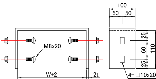
角根丸頭ボルト・ナット 4組含む
