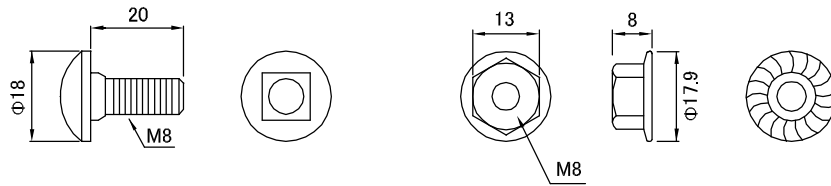
角根丸頭ボルト
